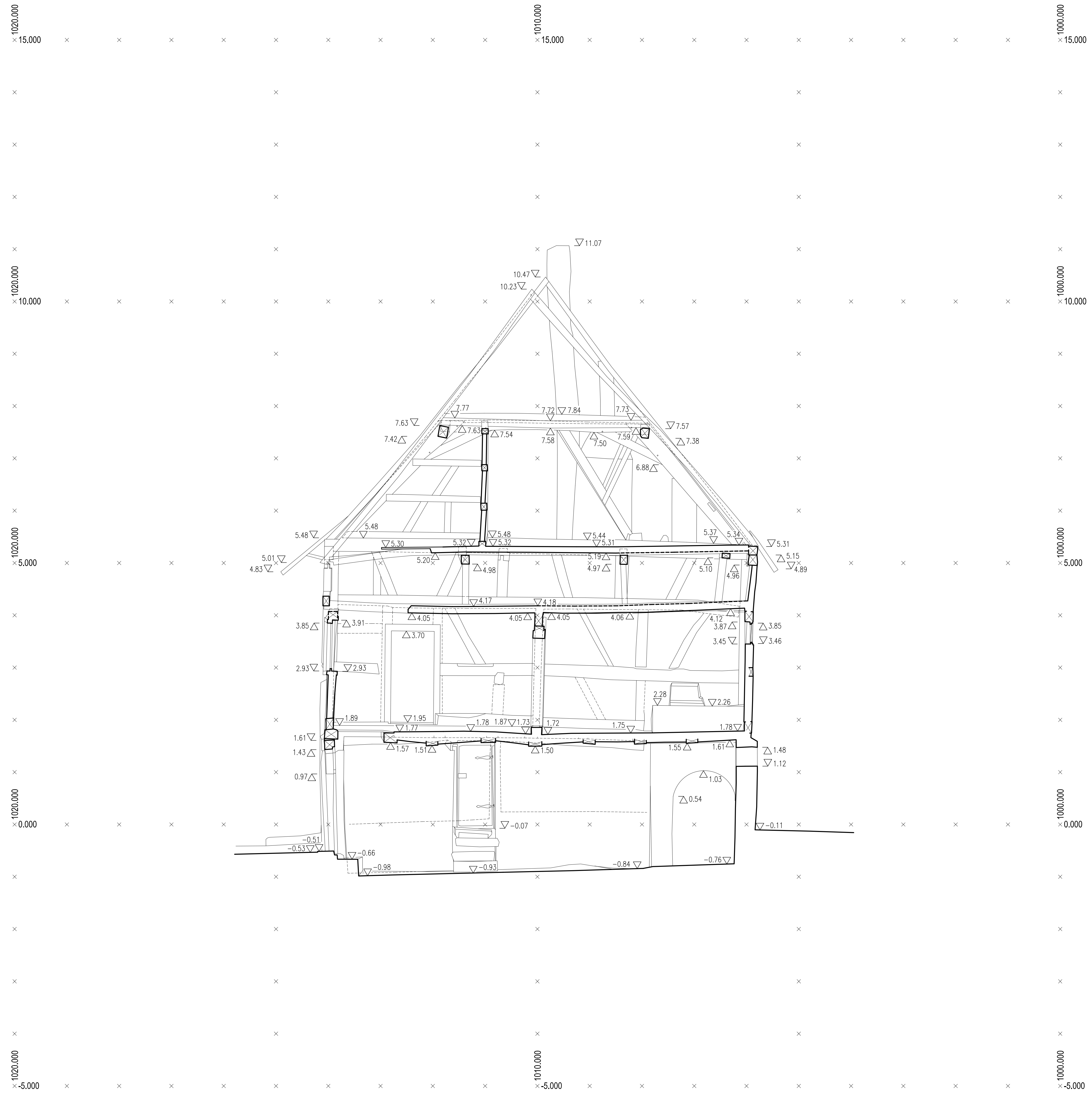
Schnitt C-C Wohnhaus – Theodor-Heuss-Strasse 51 Lachen-Speyerdorf
