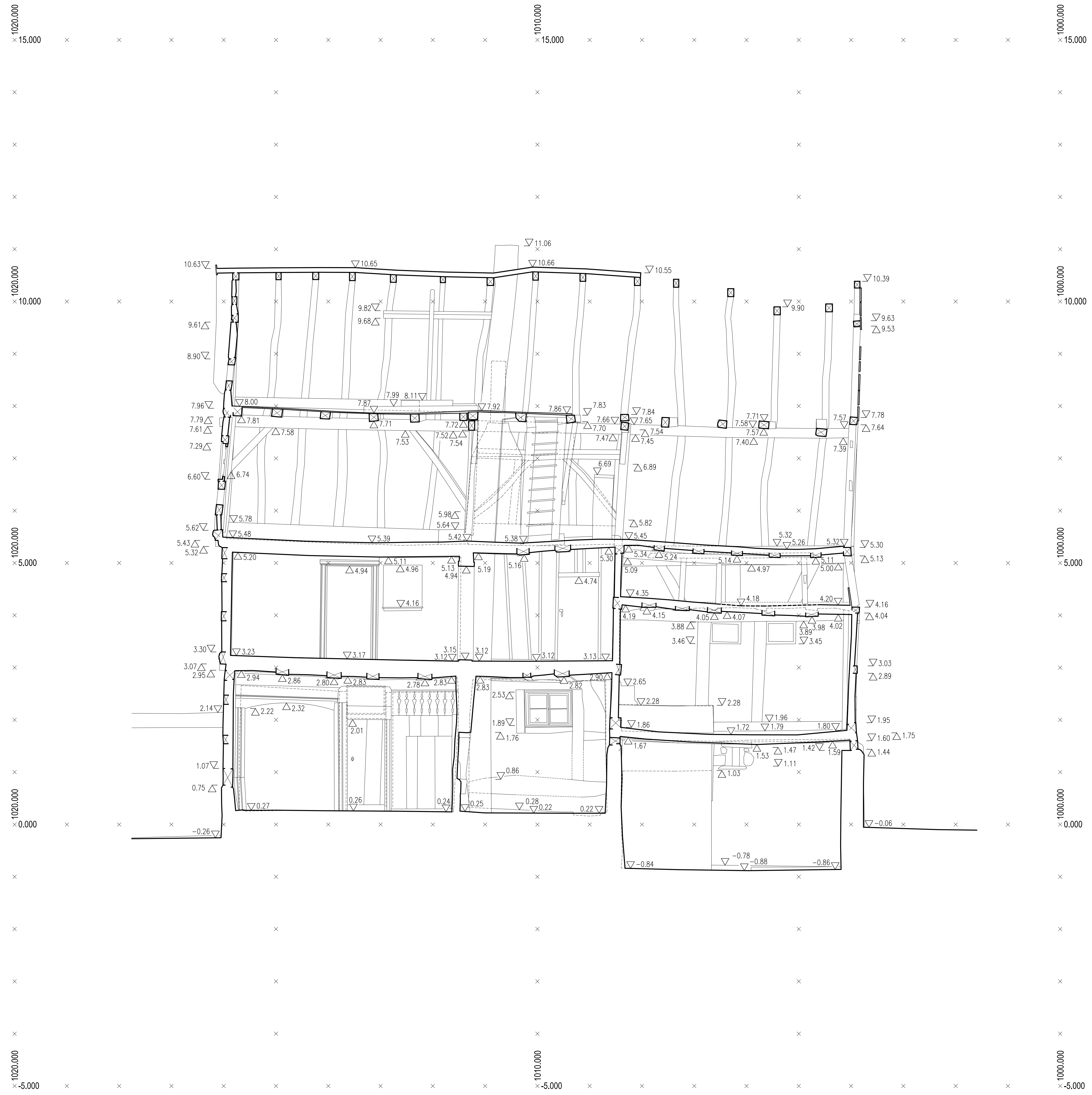
Schnitt A-A Wohnhaus – Theodor-Heuss-Strasse 51 Lachen-Speyerdorf
