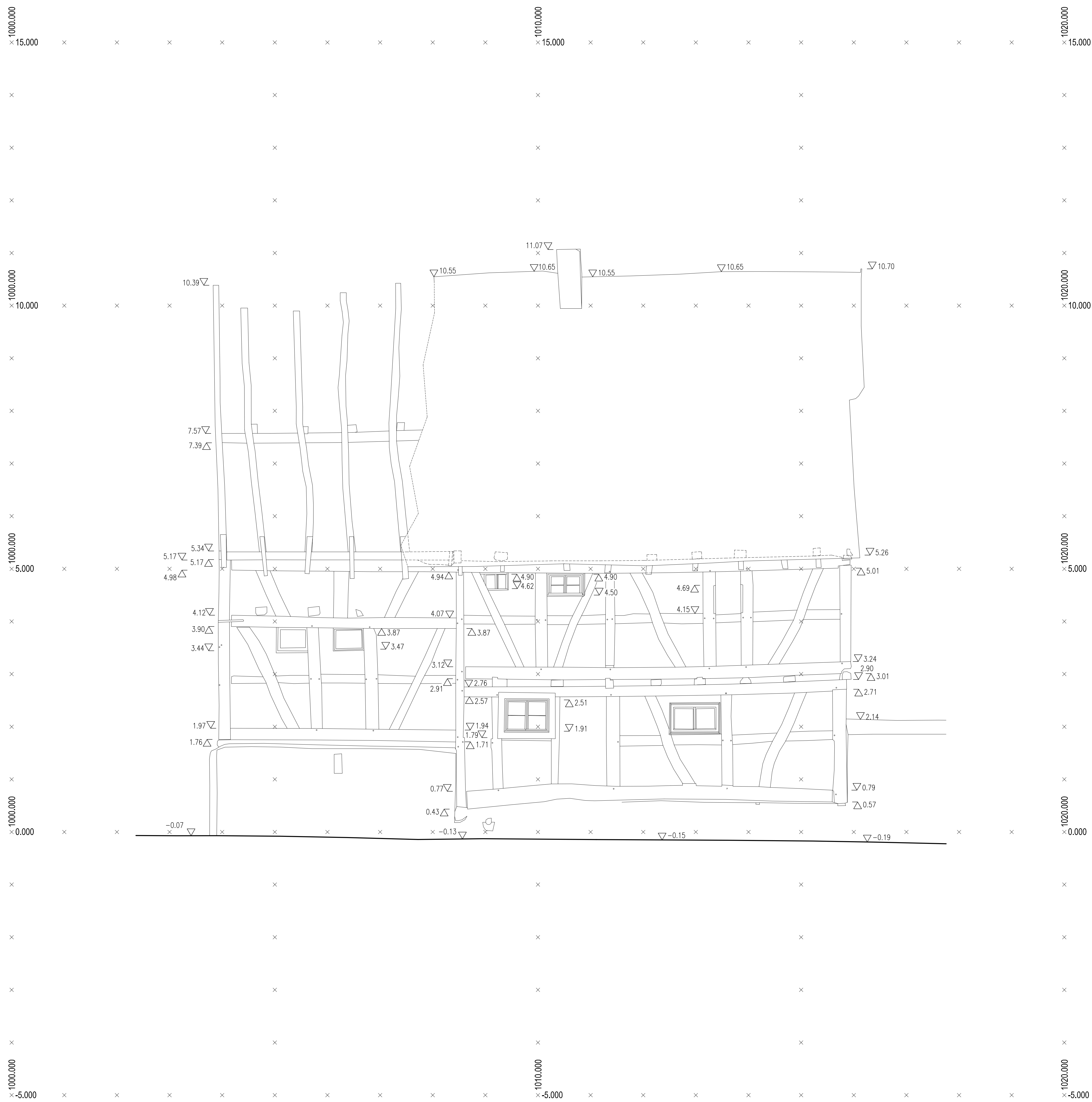
Ansicht Südwest Wohnhaus – Theodor–Heuss–Strasse 51 Lachen–Speyerdorf
